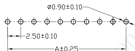
P.C.B Layout
