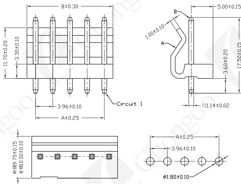
P.C.B Layout
